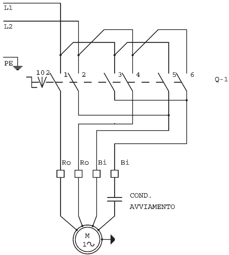
MOTORE RIDUTTORE
